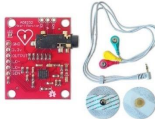
Gambar 4.6 AD8232
